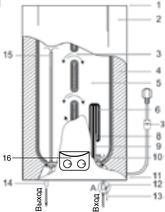
Серия FSL1/FSP1
