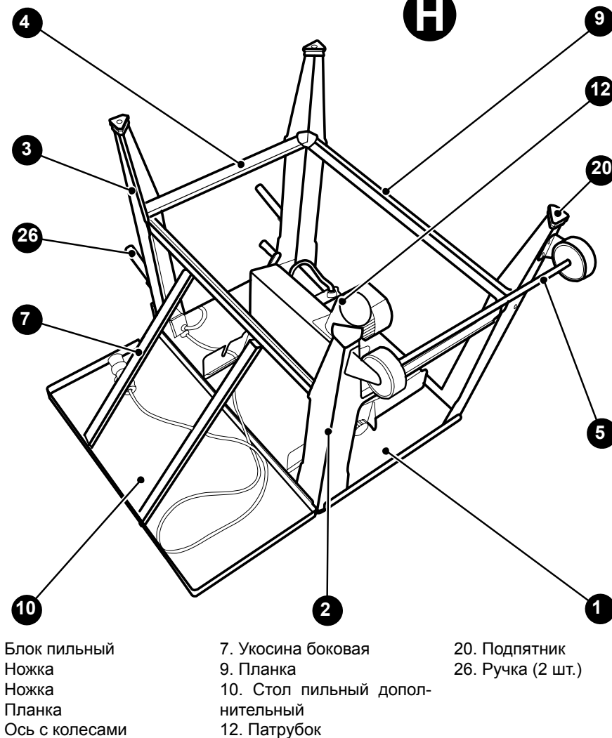
Рисунок Н — сборка станка.
