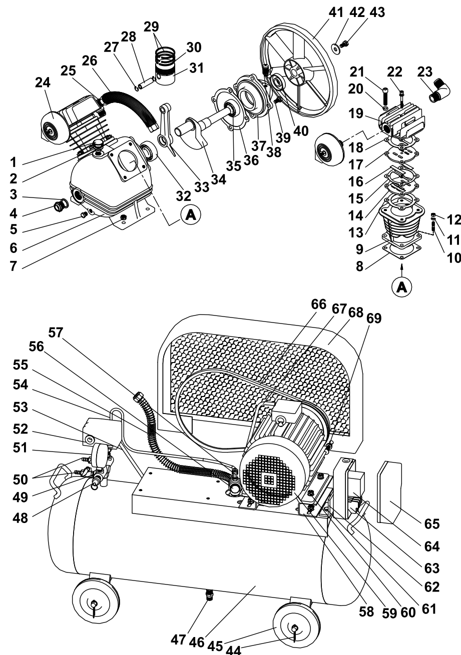
Рисунок № 1 — схема сборки компрессора.
