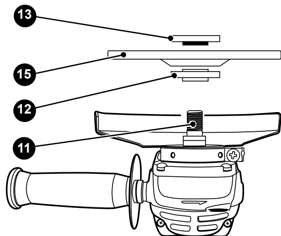
Рисунок D — установка и крепление абразивного шлифовального круга.
