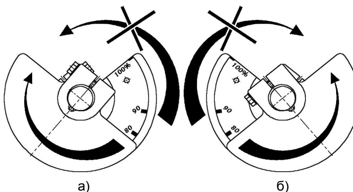
Рисунок 5. Схема регулировки статического момента плавно регулируемых дебалансов ИВ-16-100: а) на левом конце вала; б) на правом конце вала.
