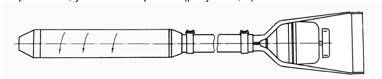
Рисунок 6. Схема установления направления вращения вала ротора вибраторов ИВ-78, ИВ-102А.
