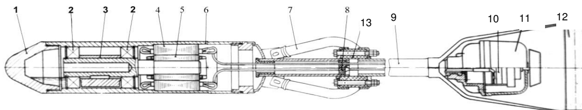
Рисунок 5. Вибратор ИВ – 103.
