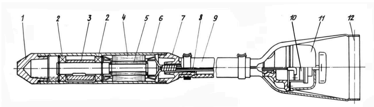
Рисунок 4. Вибратор ИВ – 102А.
