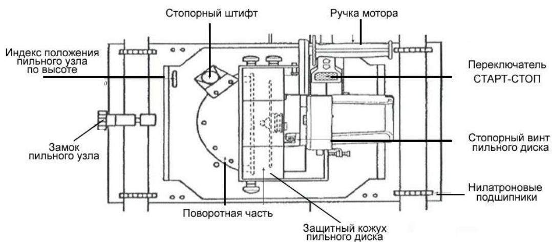
РИС. 11. Основные компоненты пильного узла (модель С4, С5, все станки серии Н)
