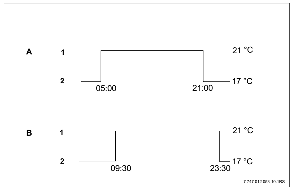
Рис. 20 Новая программа отопления
