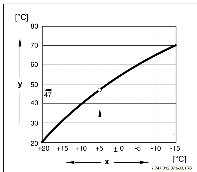
Рис. 3 Графическая характеристика отопительного контура (пример)
