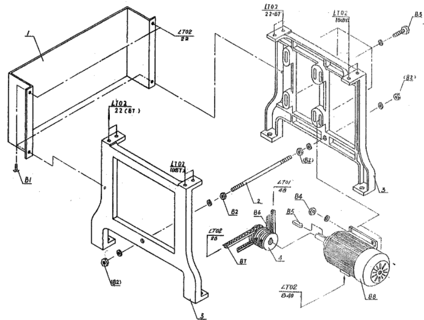
ДЕТАЛИ СБОРКИ «КОРВЕТ 321» *- позиция по схеме сборки Схема 3
