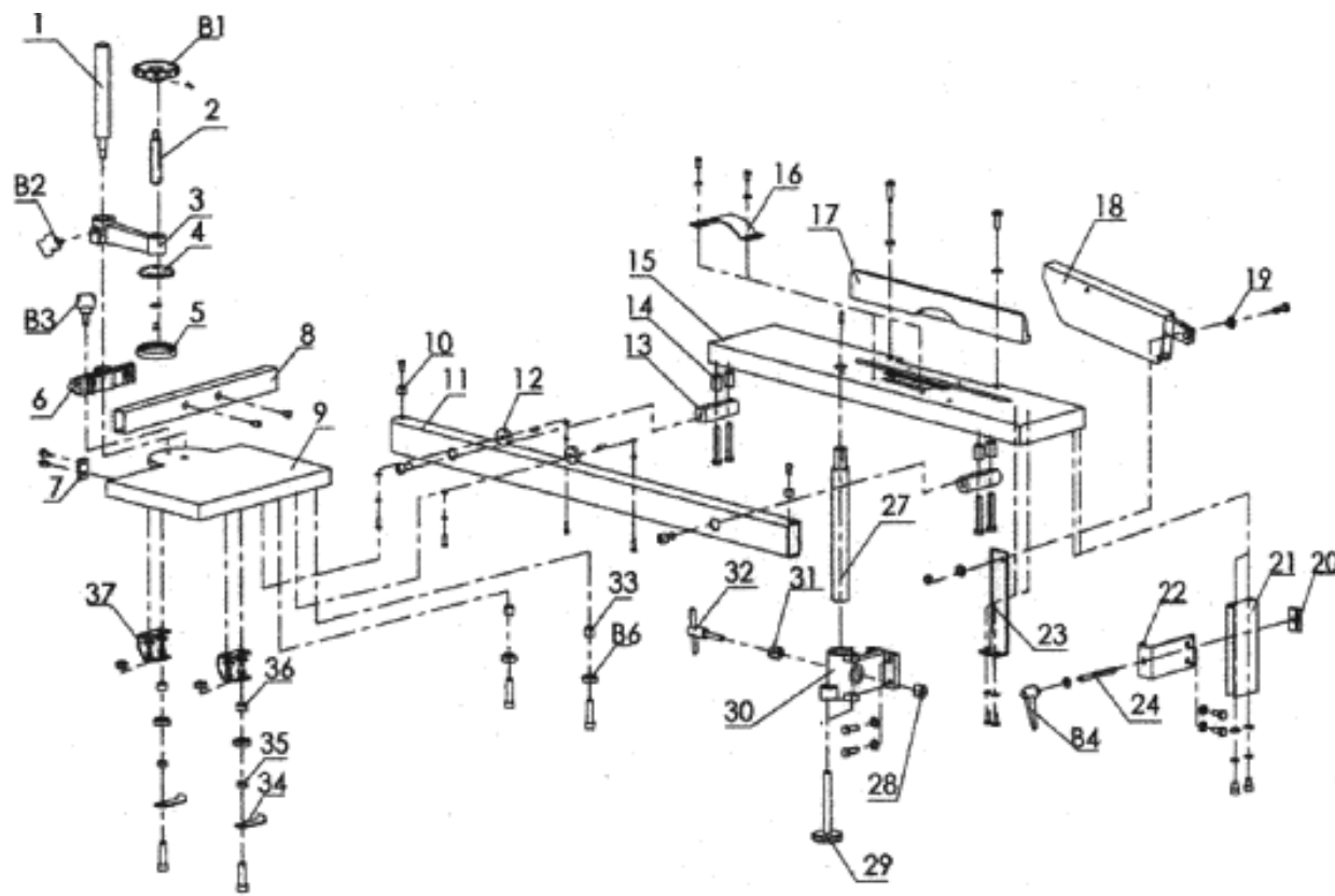
СХЕМА СБОРКИ «КОРВЕТ 321» Схема 4
