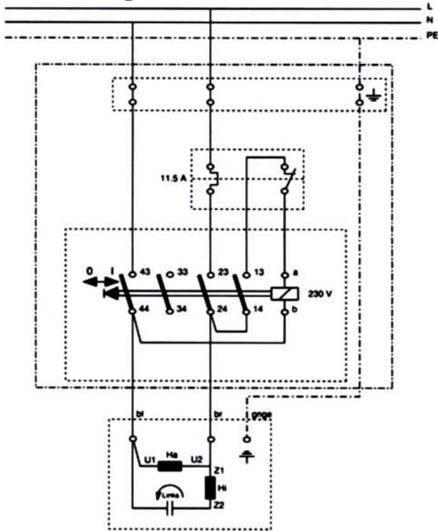
Электрическая схема станка
