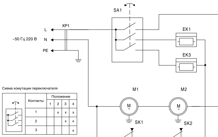
Рис. 4. Схема электрическая BHC-9.000SR
