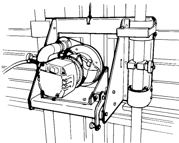
РИС. 4. Установка платформы с фрезерным мотором (показана модель 3400)
