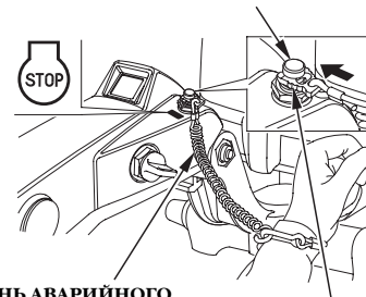
СКОБА АВАРИЙНОГО ВЫКЛЮЧАТЕЛЯ ДВИГАТЕЛЯ
