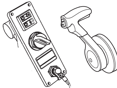
ПАНЕЛЬ ВЫКЛЮЧАТЕЛЕЙ И ОТДЕЛЬНО УСТАНОВЛИВАЕМЫЙ ПОСТ ДИСТАНЦИОННОГО УПРАВЛЕНИЯ (ДЛЯ ОДИНАРНОЙ СИЛОВОЙ УСТАНОВКИ)
