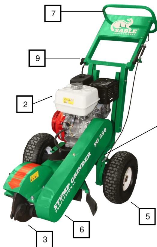
Общий вид SG 350
