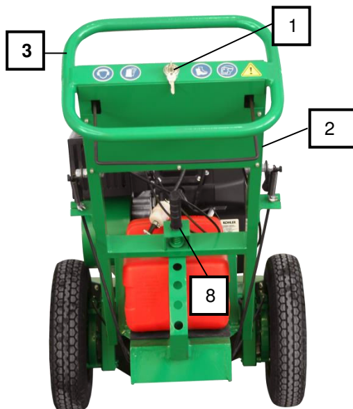
Вид панели управления SG 450 с рабочего положения
