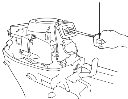
РУЧКА СТАРТЕРА
