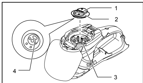
1. Veivaksel 2. Påfør smørefett. 3. Stifter 4. Forsenket sveidsl
