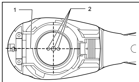
1. Grunnleggende justeringslinje på verktøyet 2. Stifter
