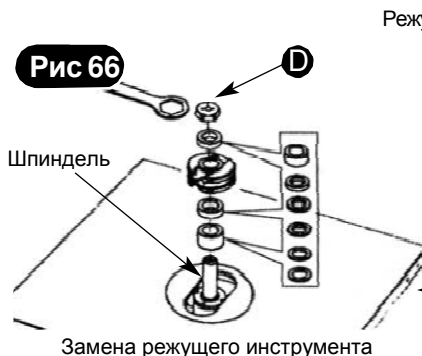
Замена режущего инструмента
