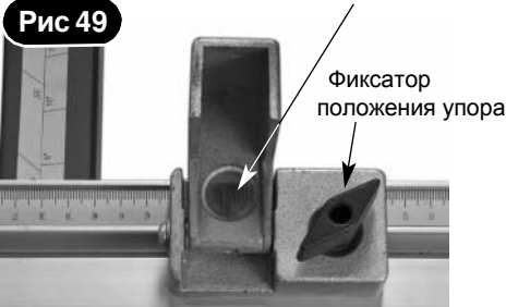
Упор установки длины фрезерования
