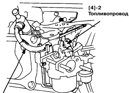
[4]-1 Высоковольтный провод
