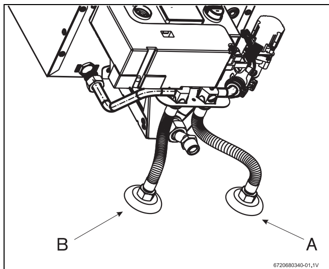
Рис 14 Подключение водопровода
