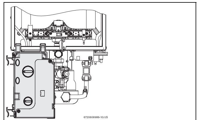
Рис 17 Блок управления – положение для регулировки подачи газа
