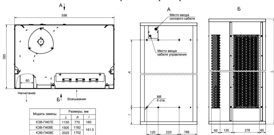
Рис. 6. Крепежные размеры
