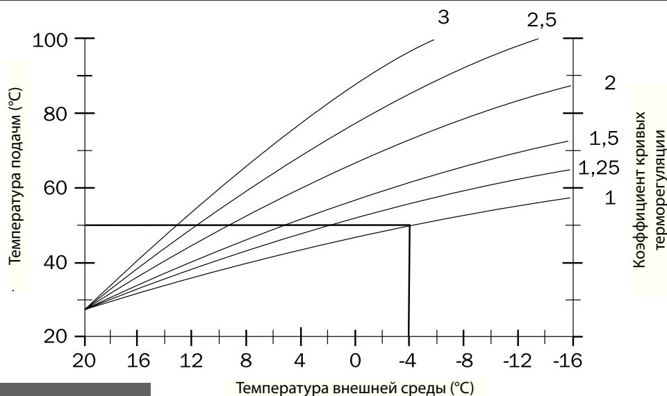
рис. 2 - Кривые терморегуляции
