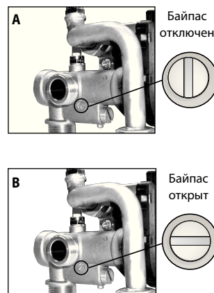
рис. 25 - Регулируемый байпас
