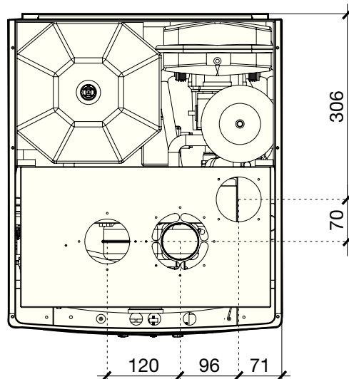
вид сверху
