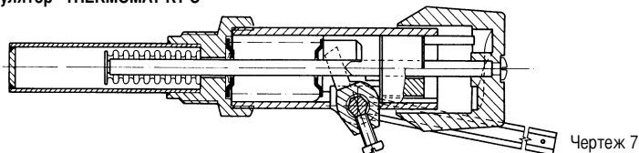
Терморегулятор "THERMOMAT RT-C"
