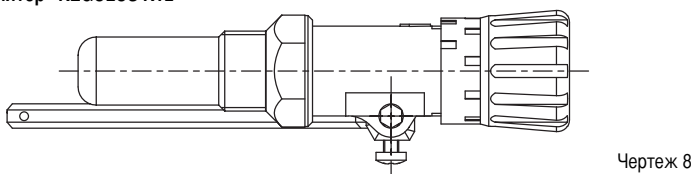
Терморегулятор "REGULUS RT2"
