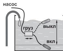
Работа на заполнение накопительной емкости
