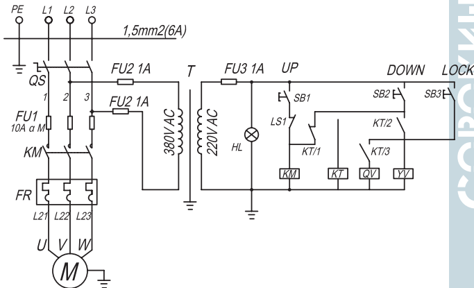
Рисунок 7а – Схема подключения мод. 17.13
