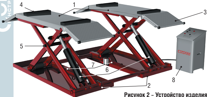
Рисунок 2 – Устройство изделия
