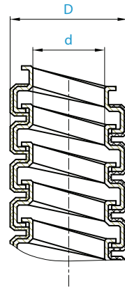
Рис. 1 - Габаритные размеры металлорукава РЗ-ЦПнг-LS
