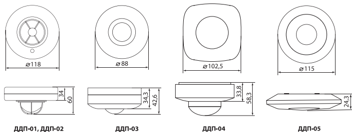
Рисунок 2. Габаритные и установочные размеры датчиков, мм
