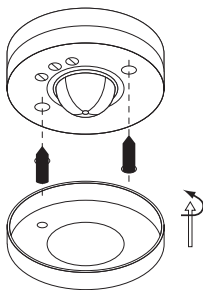
Рисунок 6. Схема монтажа датчиков ДДП-01, ДДП-02, ДДП-03, ДДП-04, ДДП-05
