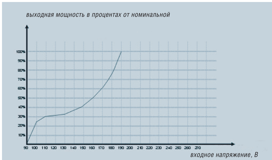
График соотношения выходной мощности и входного напряжения
