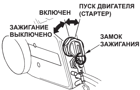
Выключатель двигателя (модификация R)
