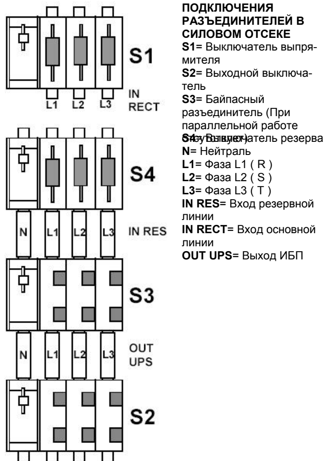
Рисунок 9D: ИБП мощностью 120-160кВА 6-пульсовой схемы и 100-120кВА 12-пульсовой схемы.
