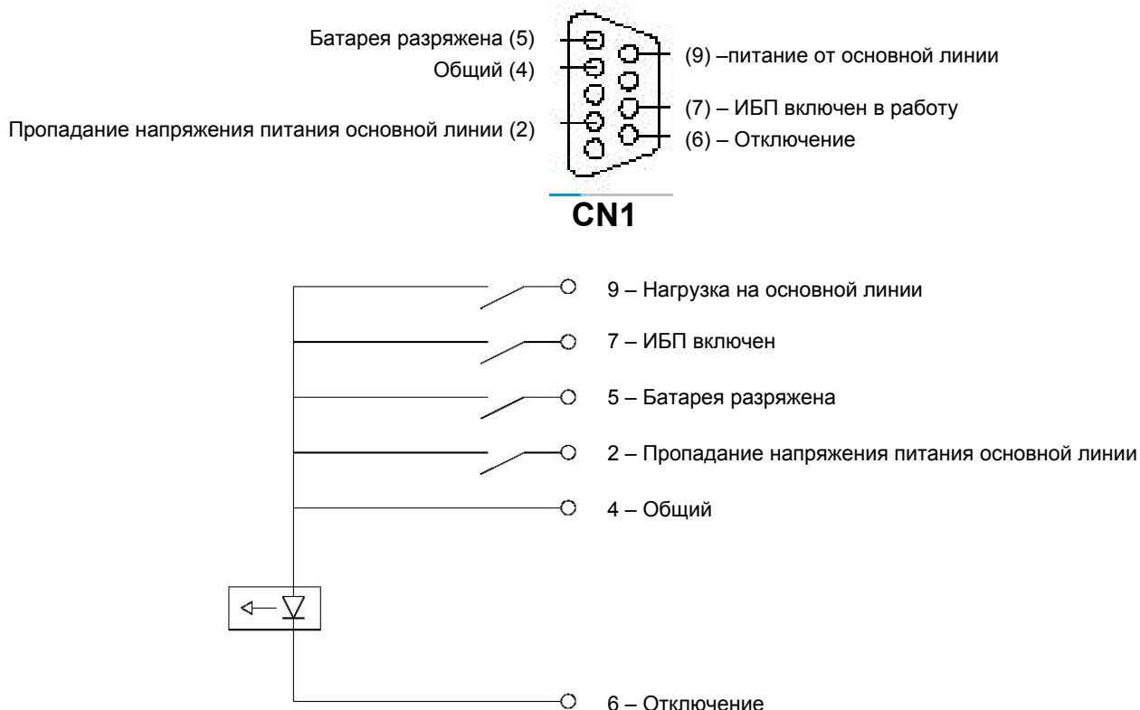
РИСУНОК 6: ПЛАТА ИНТЕРФЕЙСА ПОТРЕБИТЕЛЯ.
