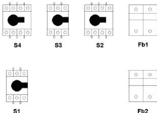
Рисунок 3А: ИБП мощностью 20-40кВА 6-пульсовой схемы и 12-пульсовой схемы.
