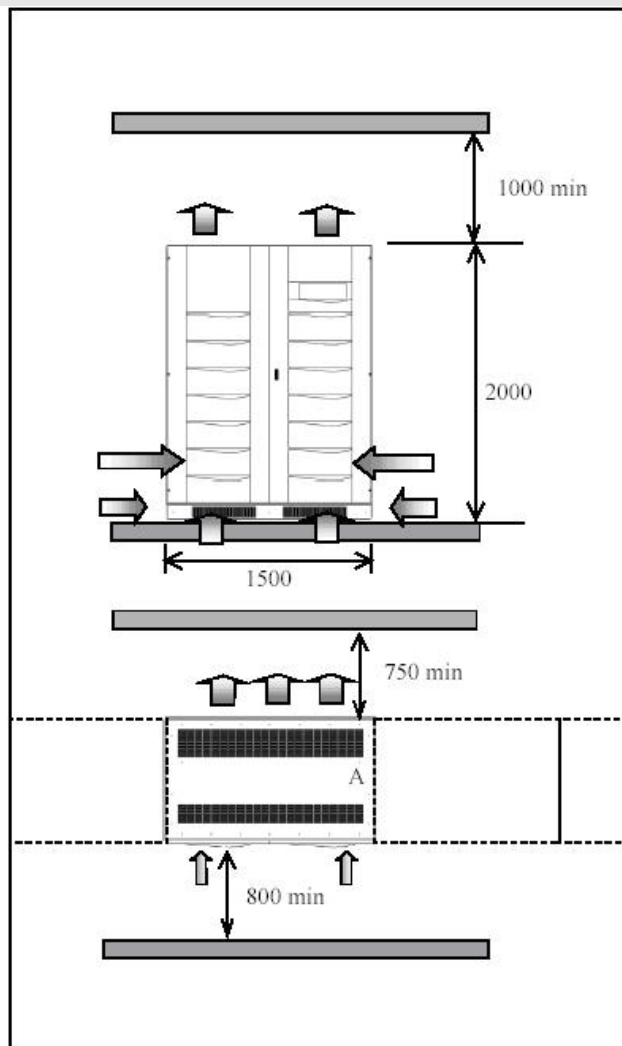
Рисунок 10Е: ИБП мощностью 250-400кВА.
