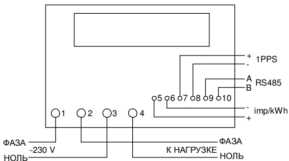
Схема подключения счётчиков НЕВА МТ 12Х
