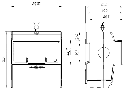
Внешний вид счётчиков НЕВА МТ 124
