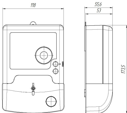
Внешний вид счётчиков НЕВА МТ 11Х
