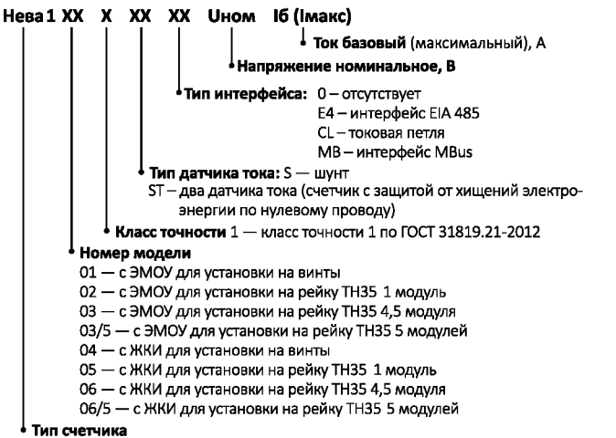
Рисунок 1. Структура условного обозначения счетчиков НЕВА 1.
