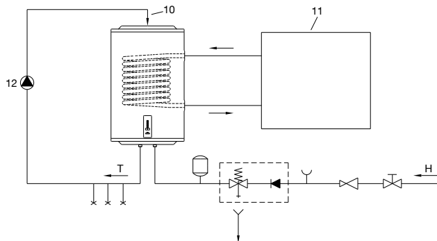
Рис. 4: Подключение водонагревателя к дополнительному источнику энергии
