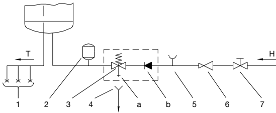
Малюнок 2: Напірна (закрита) система
