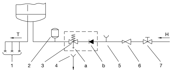
2 Сурет: Қысымды (жабық) жүйе
