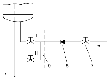
Рис. 3: Безнапорная (открытая) система
