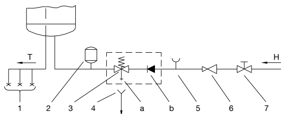
Fig. 2: Sistemul închis (presurizat)
