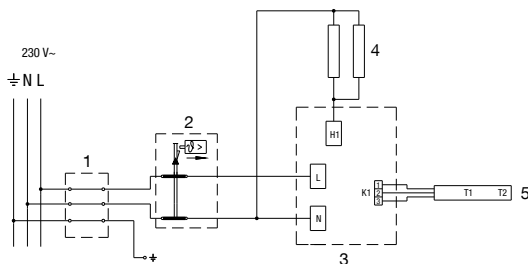
Рисунок 6: Электросхема
