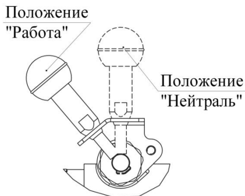
Рисунок 10 – Механизм включения косилки к мотоблоку «Угра».
