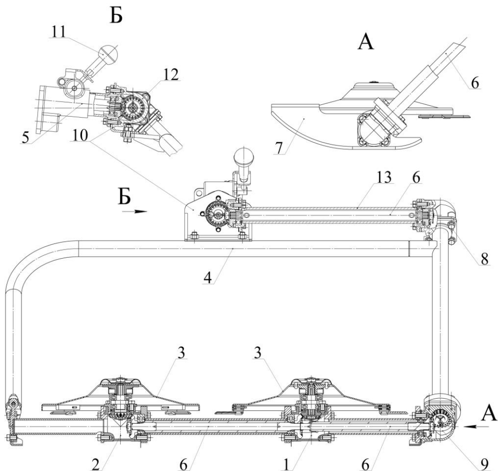
Рисунок 16 – Косилка роторная навесная «Заря» (KR.05.000-05).
