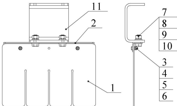
Рисунок 6 – Установка шторки на мотоблоки: «Салют», «Авангард».
