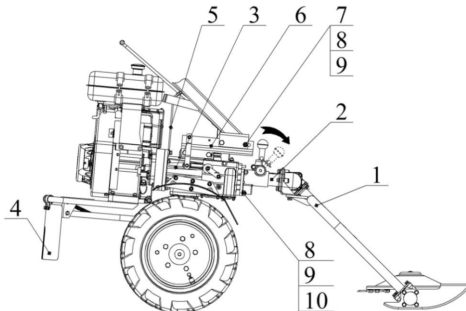
Рисунок 8 – Установка косилки на мотоблок «Угра».
