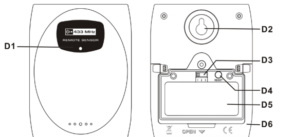
D1: Светодиод передачи сигнала D2: Отверстие для закрепления на стене D3: Переключатель номера канала
