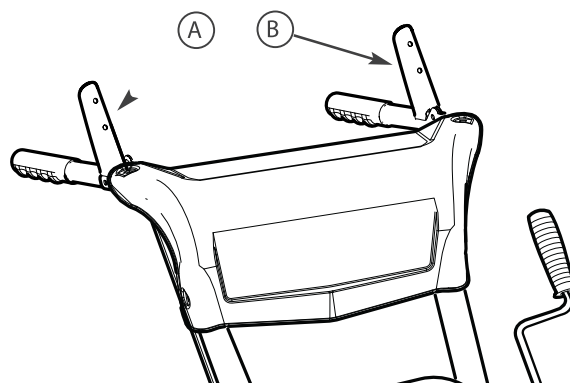
Органы управления снегоочистителем
