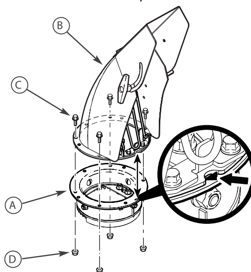
Установка разгрузочного желоба
