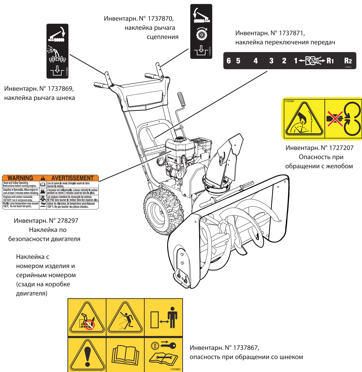
Наклейки с предупреждениями о безопасности
