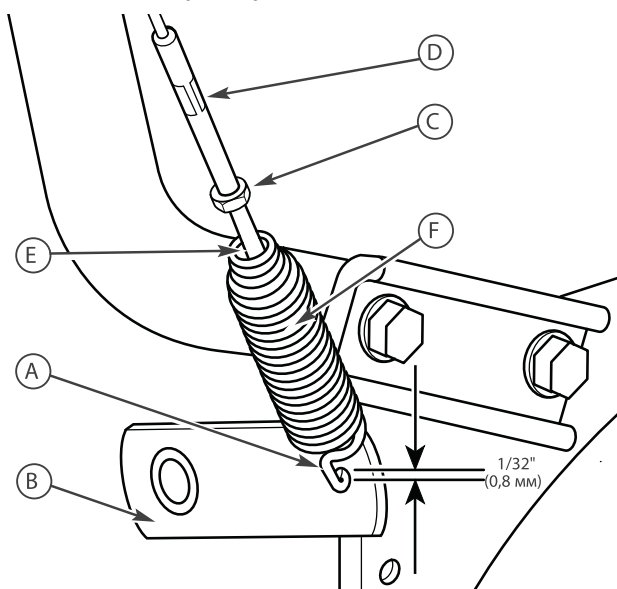
Регулировка кабеля управления шнеком
