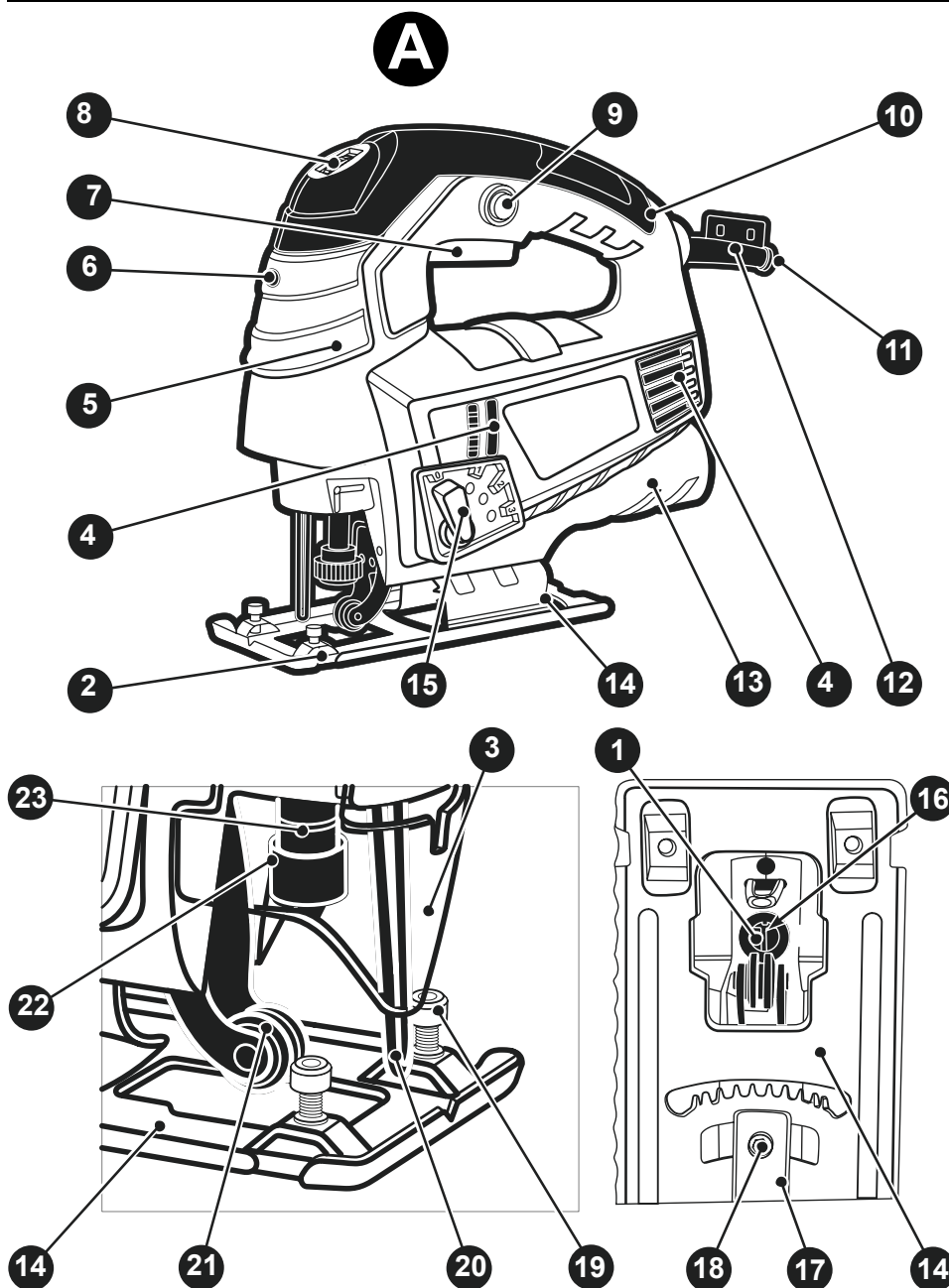
Рисунок А — общий вид лобзика.
