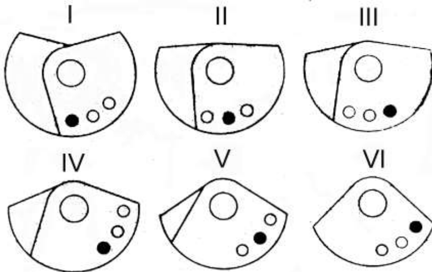
Рисунок 3. Схема регулировки статического момента
