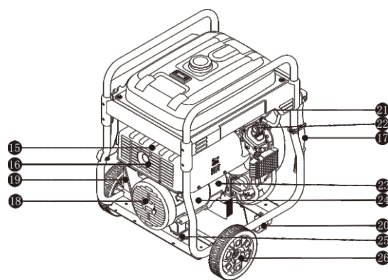
Рисунок 2. Расположение основных узлов и элементов управления.
