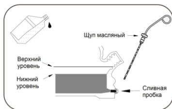
Рисунок 4. Отметки на масляном щупе.
