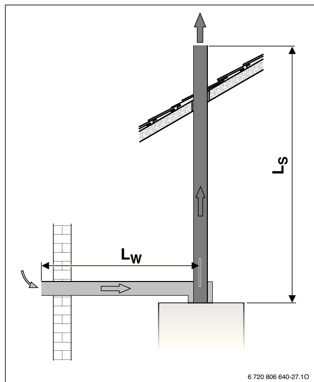
Рис. 12 Отвод дымовых газов по C_{52} с отдельной трубой
