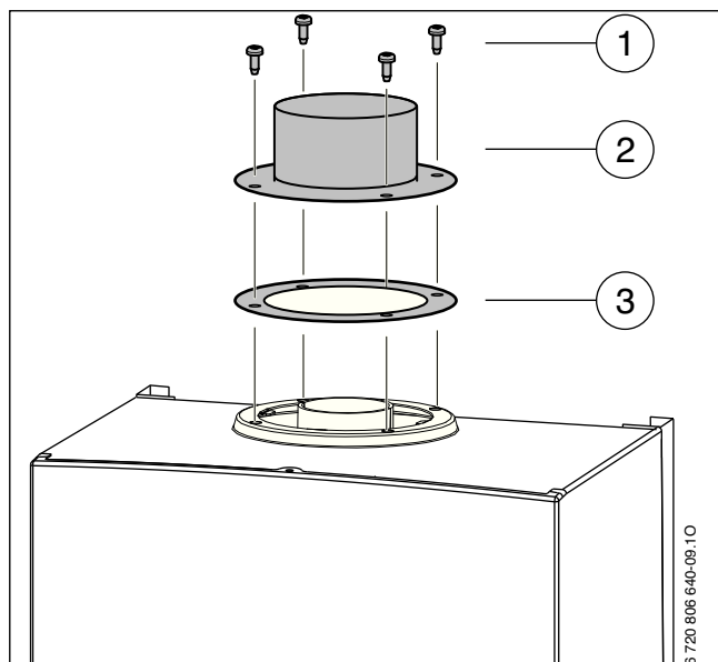
Рис. 17 Крепление переходника
