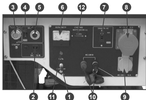
Рис. 3 Панель управления
