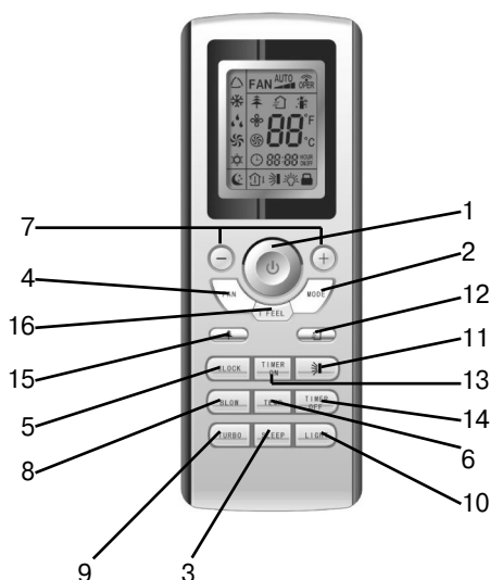
Рис. 5.1 Пульт управления
