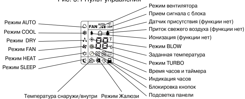
Рис. 5.1.1 Индикация пульта
