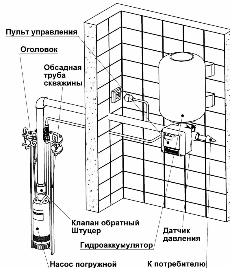
Рис.1. Система автоматического водоснабжения со скважинным погружным насосом.
