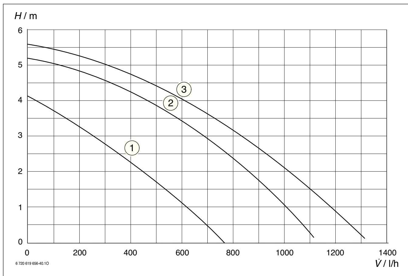
Рис. 34 Диаграмма насоса
