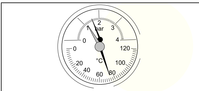
Рис. 36 Термоманометр
