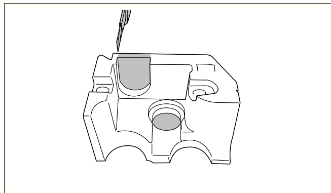
Рис. 48 Вырезание изоляции
