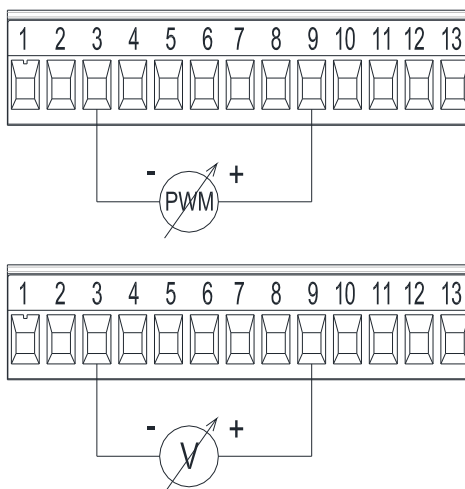
Kuv. 7: 13-napainen ulosvedettävä riviliitin: tulot 0-10V ja PWM
