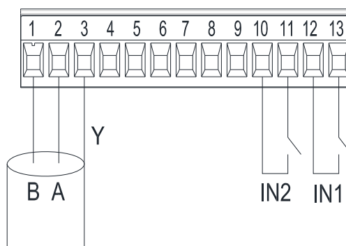
Fig. 6: 13-polig utdragbar kopplingsplint: Digitala ingångar och MODBUS
