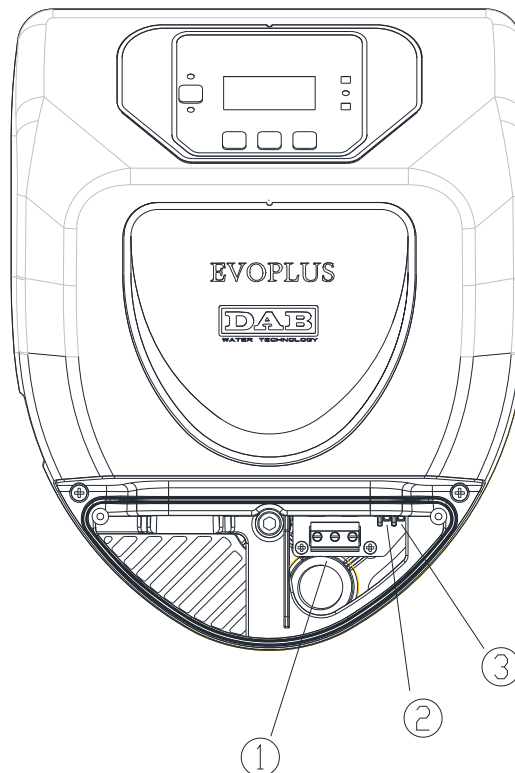
Kuv. 3: Sähköliitännät (etu)
