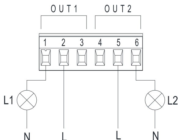
Kuv. 8: 6-napainen ulosvedettävä riviliitin: esimerkki lähtöjen kytkennästä
