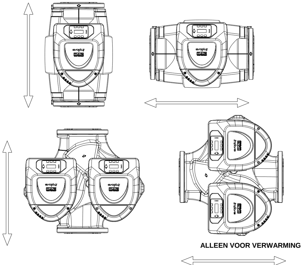
Afbeelding 1: montagepositie
