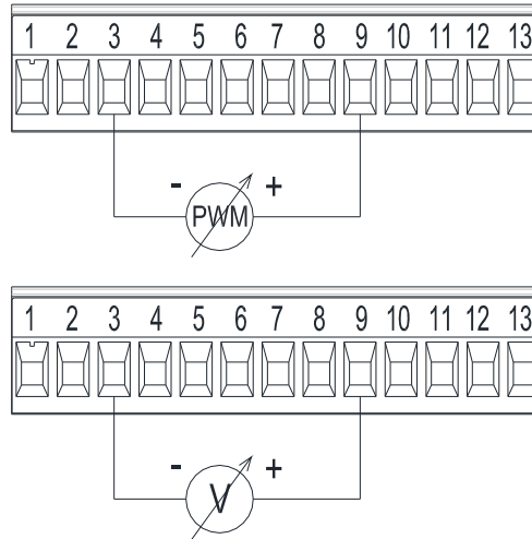
Resim 7: 13 kutuplu ekmeceli klemens kutusu: 0-10V giriřleri ve PWM
