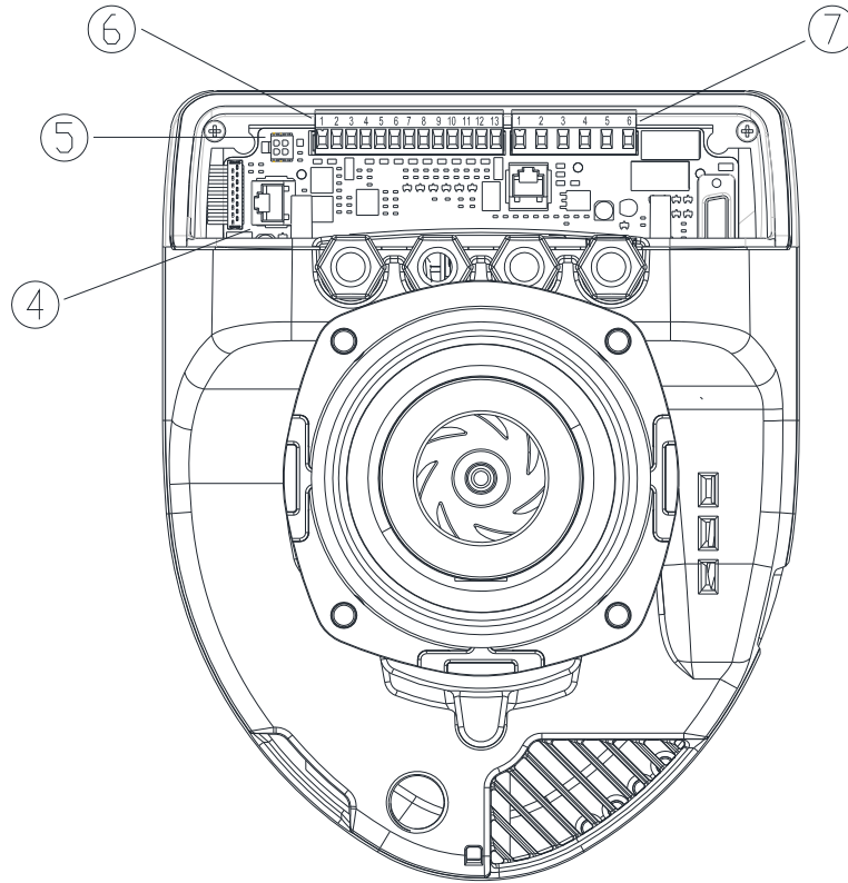
Kuv. 4: Sähköliitännät (taka)
