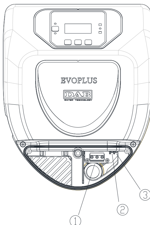
Fig. 3: Elanslutning (framsida)
