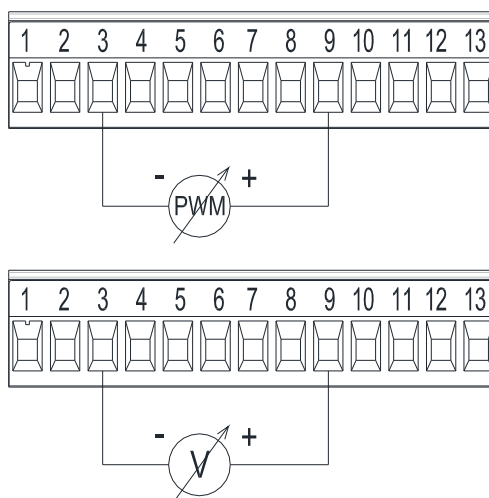
Сх. 7: Съёмная клеммная колодка 13 полюсов: входы 0-10 В и ШИМ
