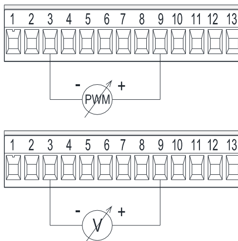
Εικόνα 7: Αφαιρούμενη κλέμμη 13 πόλων: είσοδοι 0-10V και PWM
