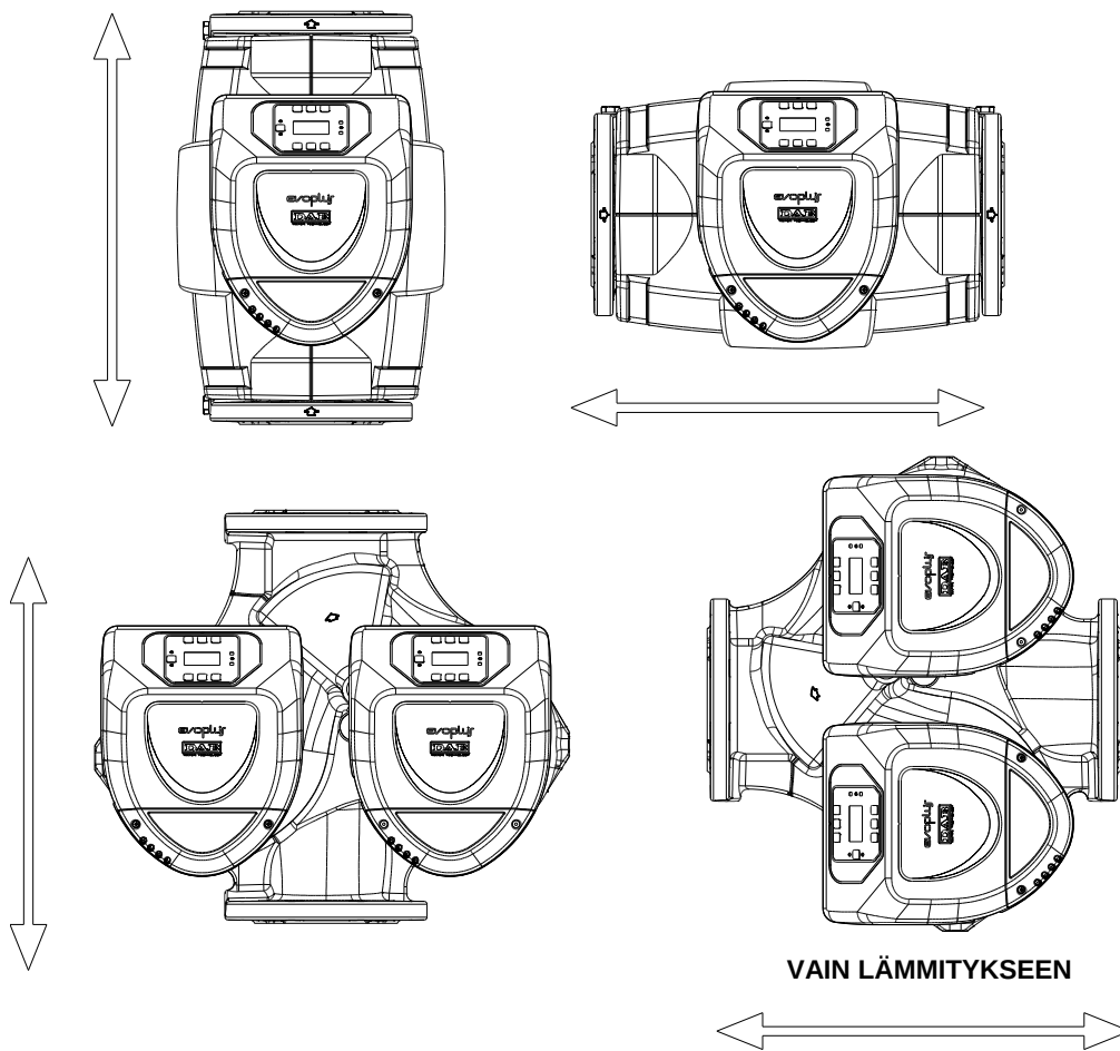
Kuv. 1: Asennusasento
