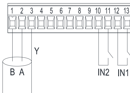
Kuv. 6: 13-napainen ulosvedettävä riviliitin: digitaaliset tulot ja MODBUS
