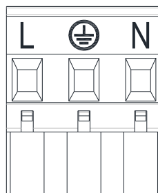
Kuv. 5: Irrotettava riviliitin
