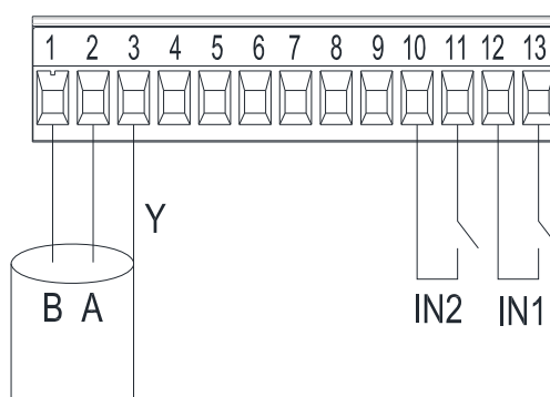
Εικόνα 6: Αφαιρούμενη κλέμμα 13 πόλων: ψηφιακές είσοδοι και MODBUS
