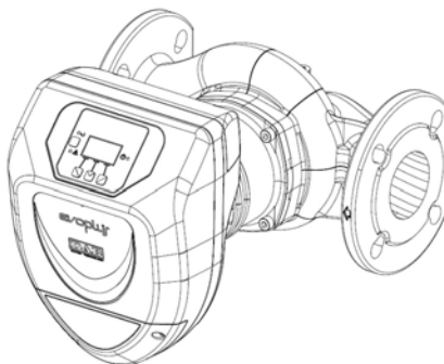
Kuv. 2: Asentaminen vaakasuuntaisiin putkiin
