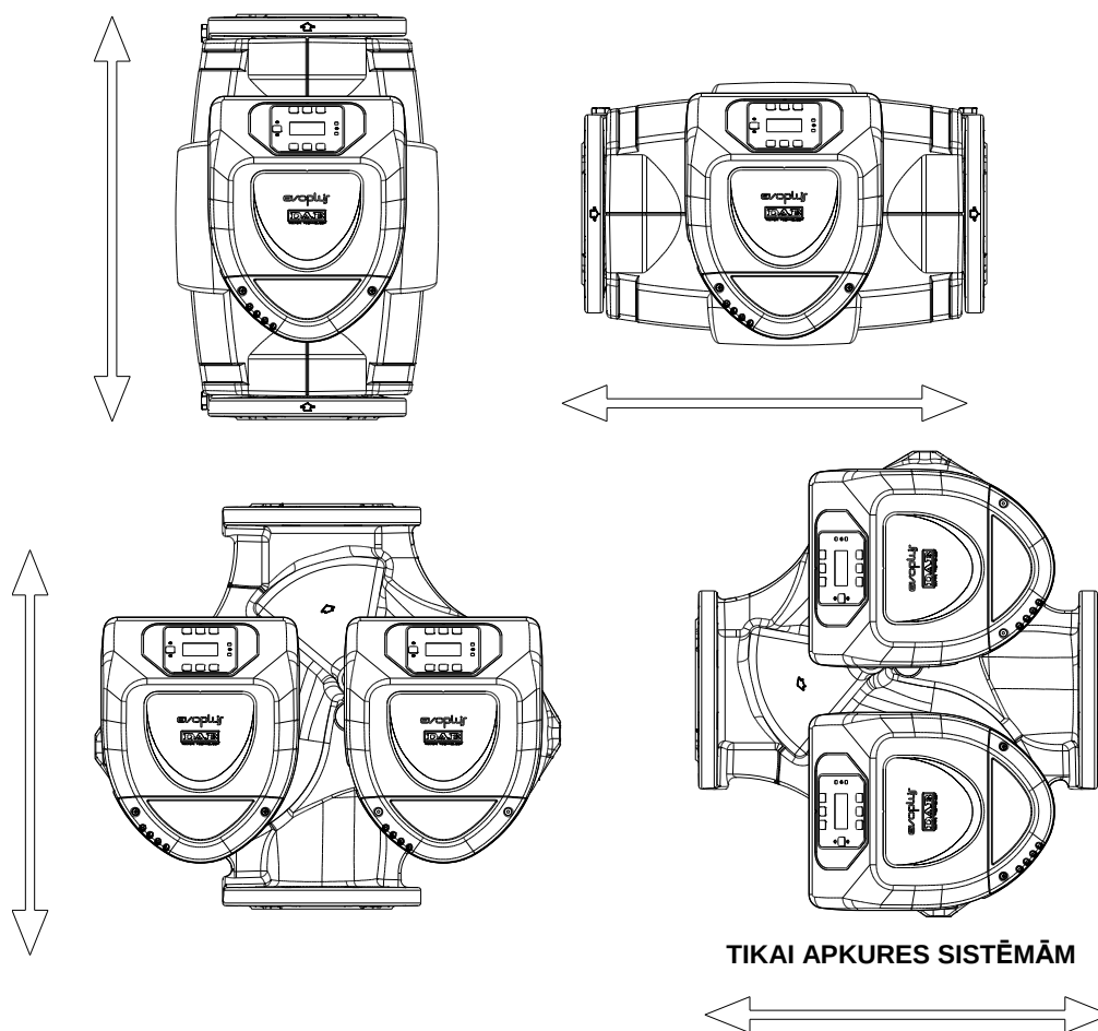
Attēls 1: Montāžas pozīcija
