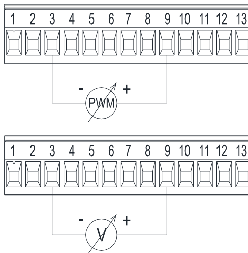
Obr. 7: Vyjímatelná 13 pólová svorkovnice: vstupy 0-10V a PWM
