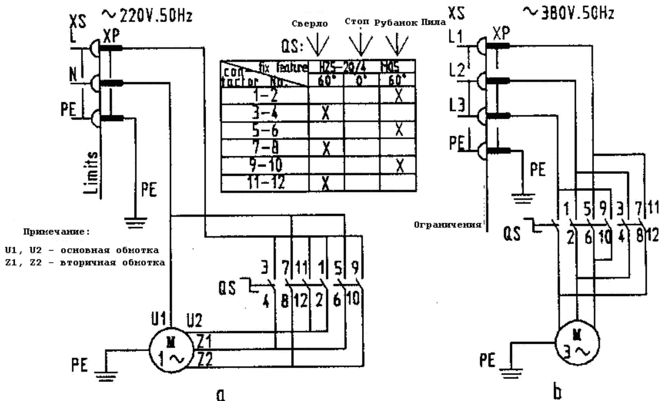
Рис.6 Электрическая схема
