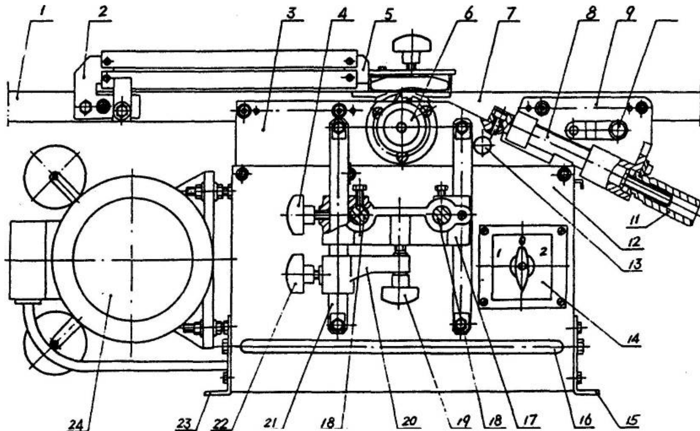
Рис. 1 Схема станка
