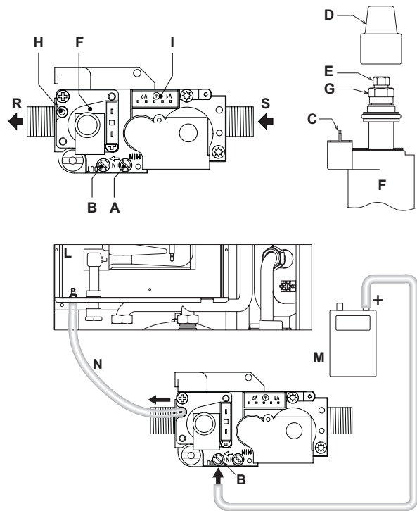
рис. 27 - Газовый клапан
