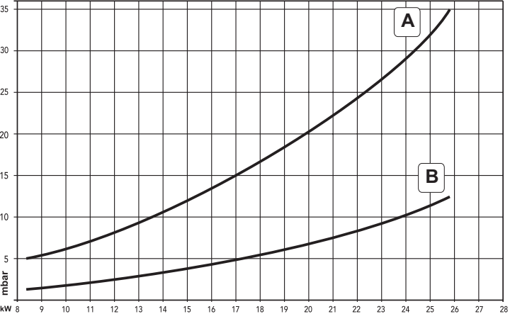
мал. 33 - Діафрагма тиску/потужність DIVAtop MICRO F 24 A GPL (зріджений нафтовий газ) B МЕТАН
