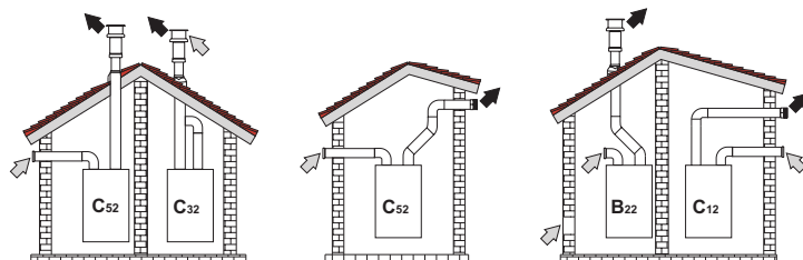
fig. 23 - Exemples de raccords avec conduits séparés (→ = Air / → = Fumées)
