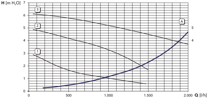
мал. 36 - Утрати напору / тиску циркуляційних насосів DIVAtop MICRO F 32 A Утрати напору у котлі 1 - 2 - 3 Швидкість циркуляційної насосу
