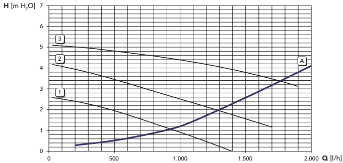
şek. 34 - Sirkülatör yük / basınç kayıpları DIVAtop MICRO F 24
