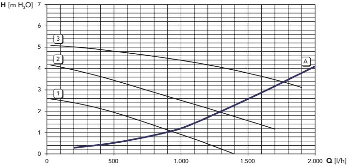
мал. 34 - Утрати напору / тиску циркуляційних насосів DIVAtop MICRO F 24 A Утрати напору у котлі 1 - 2 - 3 Швидкість циркуляційної насосу
