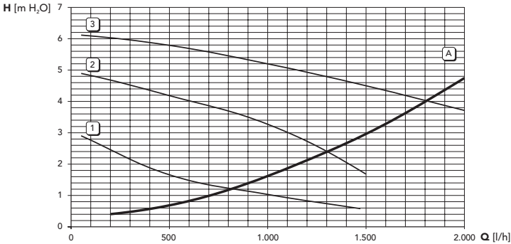
мал. 38 - Утрати напору / тиску циркуляційних насосів DIVAtop MICRO F 37 A Утрати напору у котлі 1 - 2 - 3 Швидкість циркуляційної насосу
