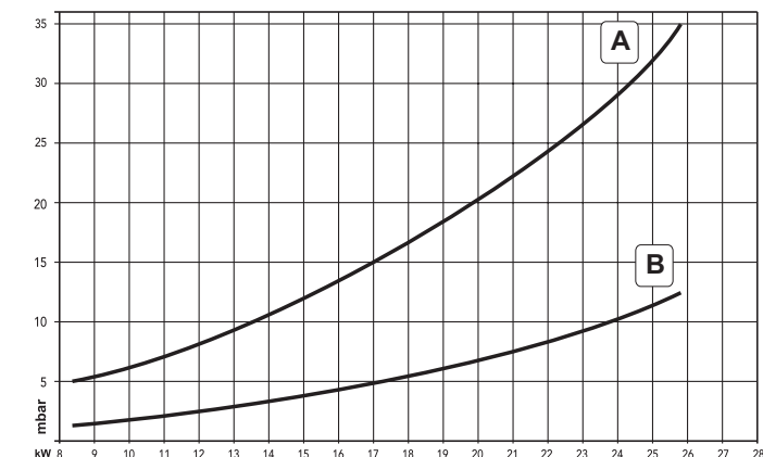
fig. 33 - Diagramma pressione/potenza DIVAtop MICRO F 24
