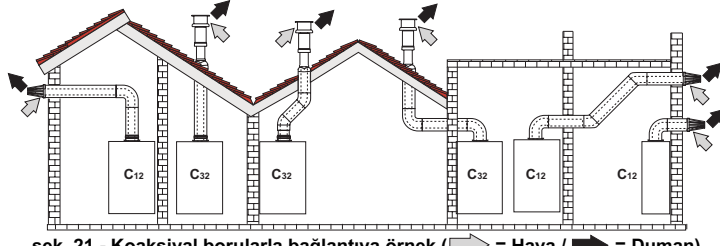
şek. 21 - Koaksiyal borularla bağlantıya örnek (→ = Hava / → = Duman)
