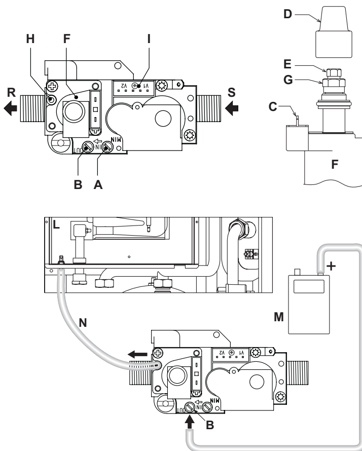
fig. 27 - Vanne à gaz
