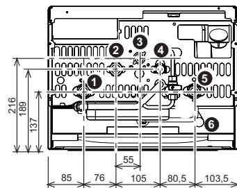
мал. 17 - Гідротехнічні підключення
