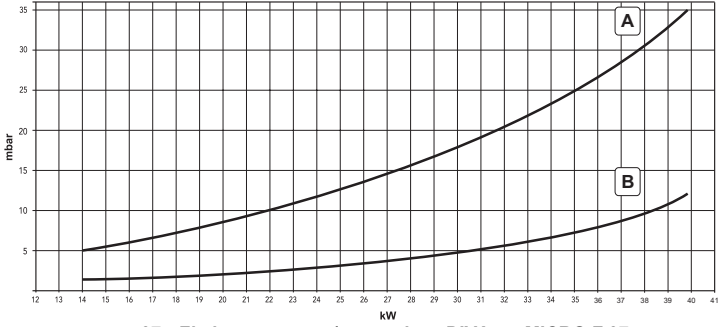
мал. 37 - Діафрагма тиску/потужність DIVAtop MICRO F 37 A GPL (зріджений нафтовий газ) B МЕТАН
