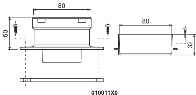
fig. 24 - Accesoriu de plecare pentru conducte separate
