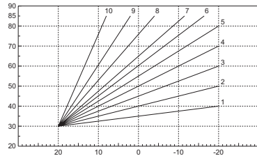
мал. 14 - Компенсаційна крива
