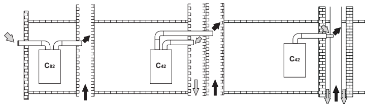
fig. 25 - Exemples de raccords à l'aide de tuyaux coaxiaux (→ = Air / → = Fumées)
