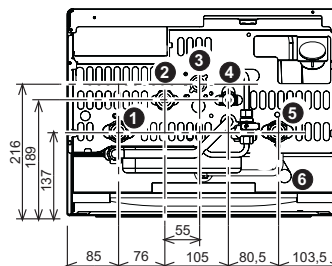
fig. 17 - Racordurile hidraulice
