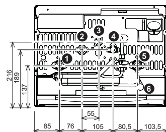
fig. 17 - Attacchi idraulici
