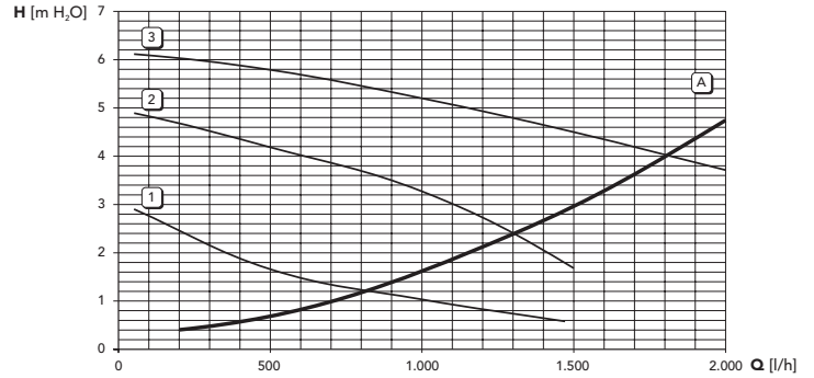
şek. 38 - Sirkülatör yük / basınç kayıpları DIVAtop MICRO F 37
