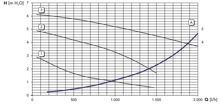
şek. 36 - Sirkülatör yük / basınç kayıpları DIVAtop MICRO F 32
