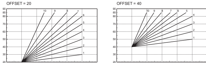
fig. 15 - Esempio di spostamento parallelo delle curve di compensazione
