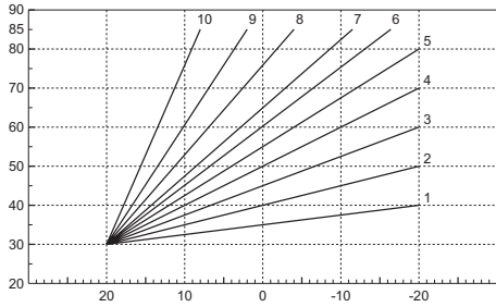
fig. 14 - Curvas de compensación
