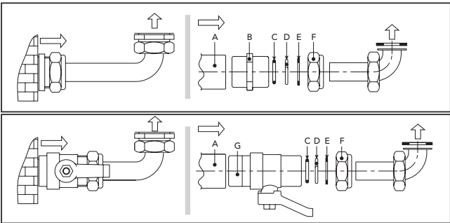
рис. 18 - Соединительный комплект
