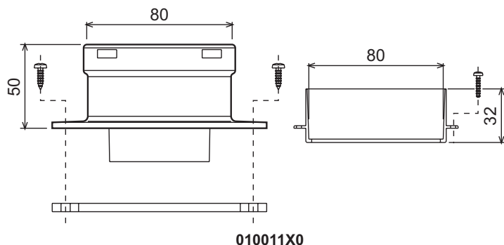
fig. 24 - Accessorio di partenza per condotti separati
