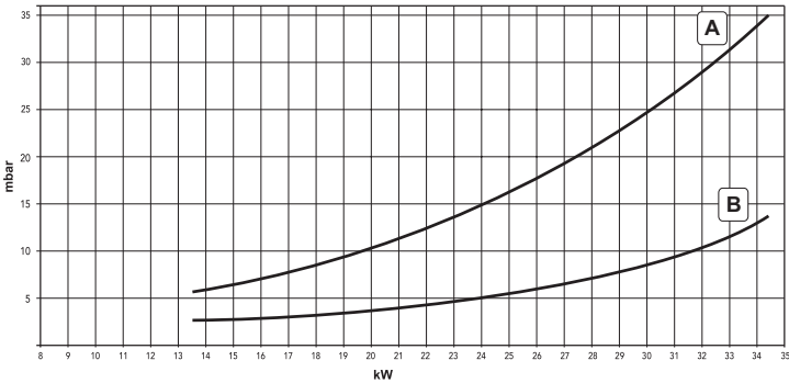
мал. 35 - Діафрагма тиску/потужність DIVAtop MICRO F 32 A GPL (зріджений нафтовий газ) B МЕТАН
