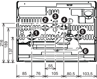
рис. 17 - Гидравлические соединения
