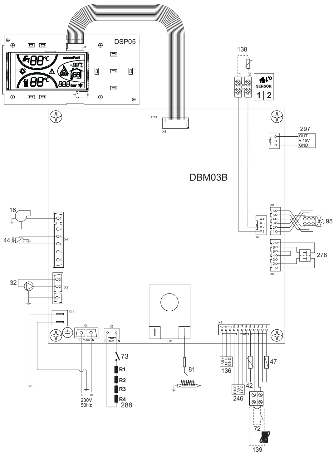
fig. 39 - Wiring diagram
